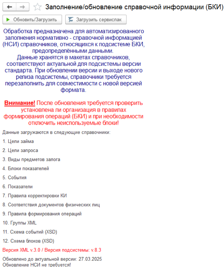
Рис. 24 – Обработка «Заполнение/обновление справочной информации (БКИ)».
