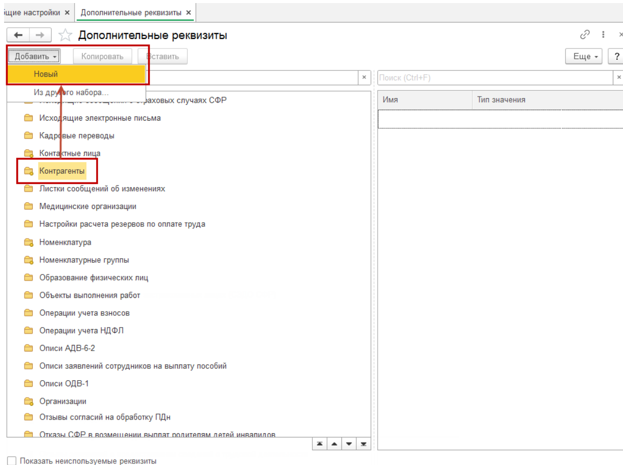
Рис. 67 – Дополнительные реквизиты.
