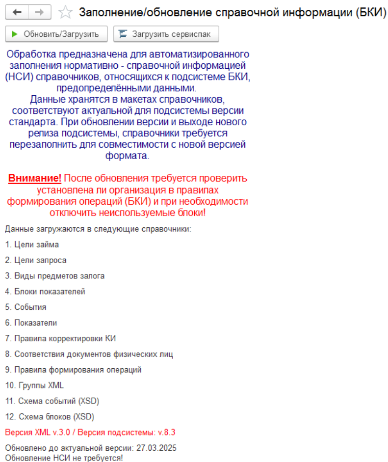
Рис. 37 – Обработка «Заполнение/обновление справочной информации (БКИ)».
