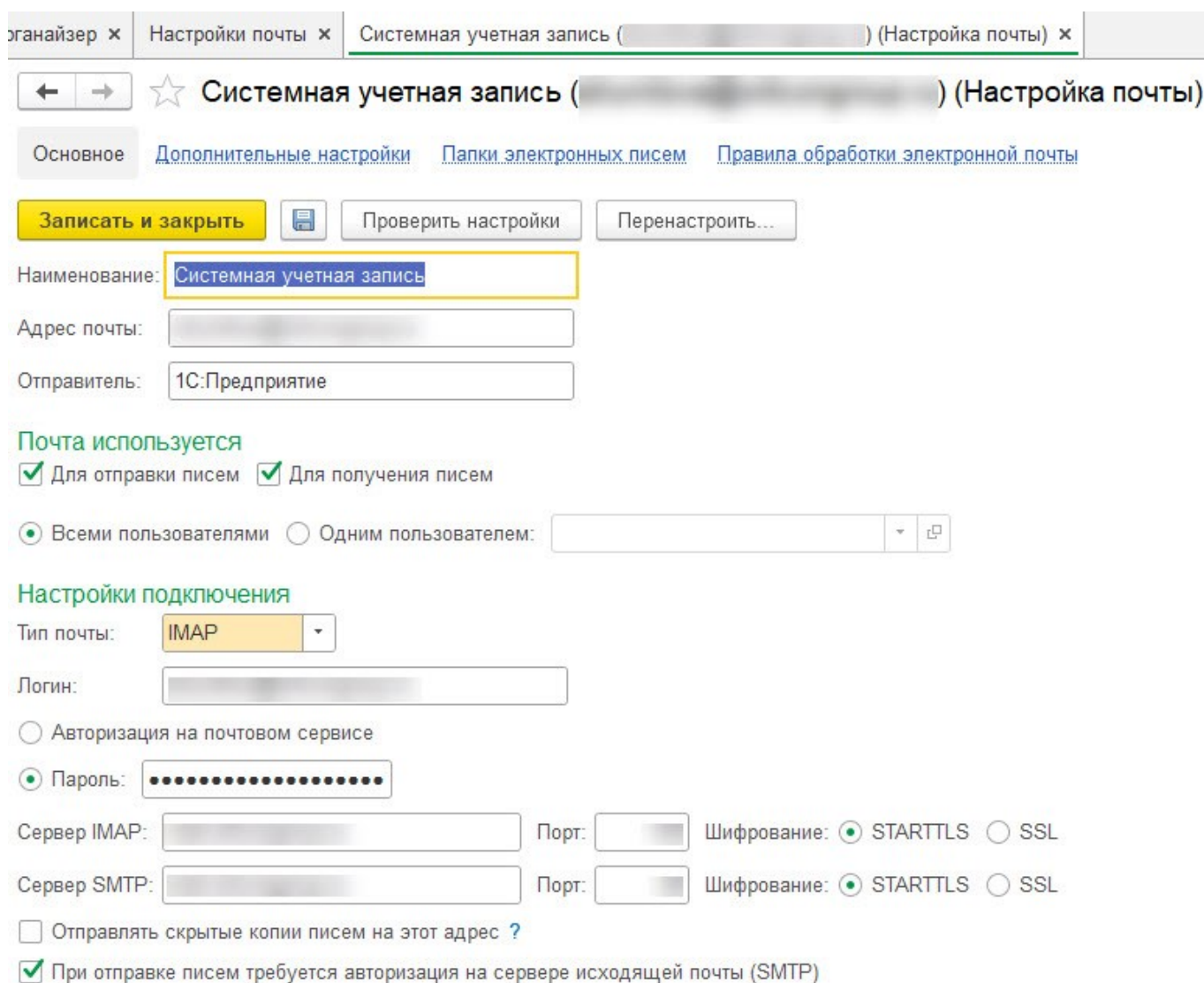
Рис. 80 – Готовый вариант настройки почты.
