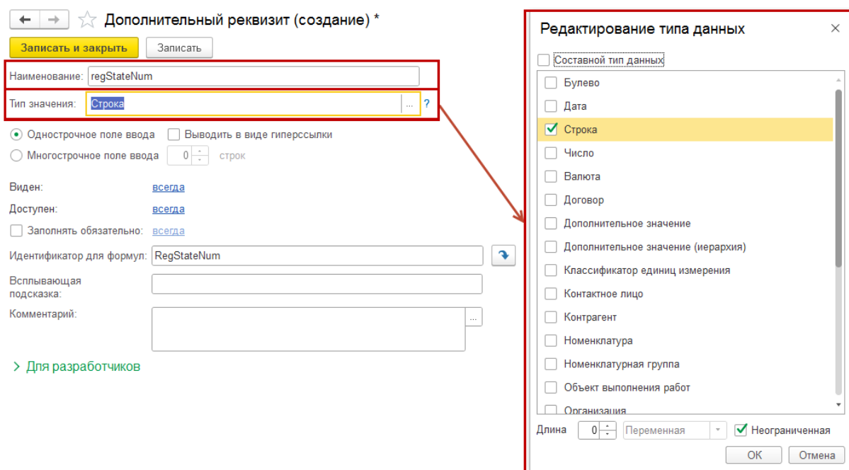
Рис. 84 – Создание дополнительных реквизитов.
