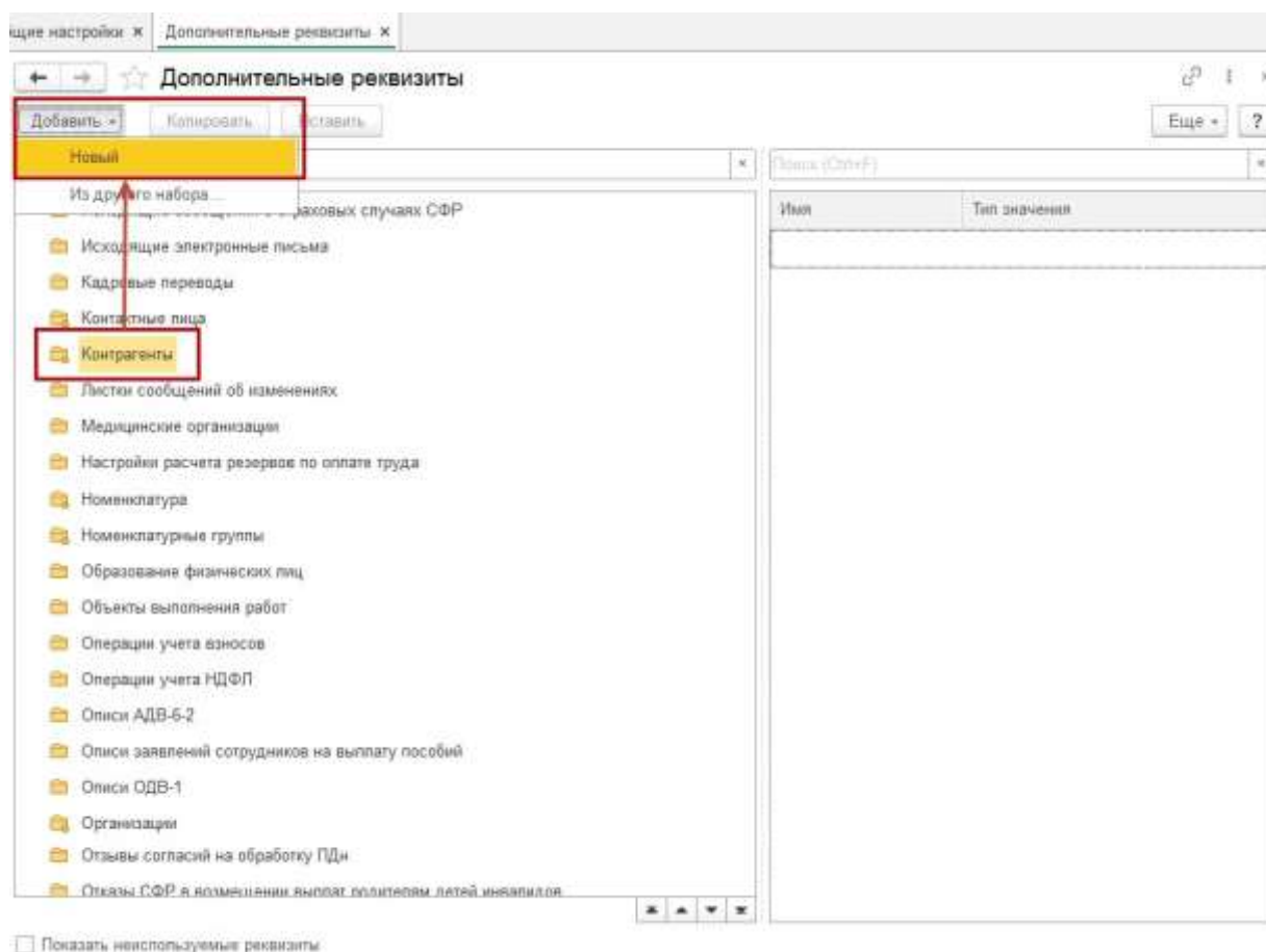
Рис. 73 – Дополнительные реквизиты.
